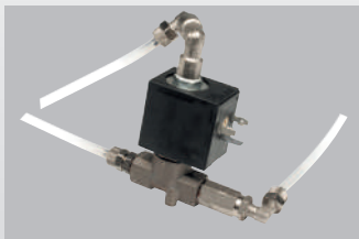
Électrovanne de mélange garantissant des températures différenciées et optimales pour les solubles
